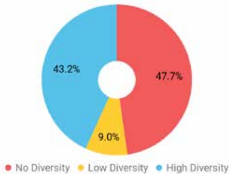
MHC Class II - DLA DRB1 CHROMOSOME 12
